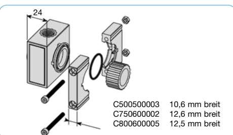
Verzweigungsplatte
