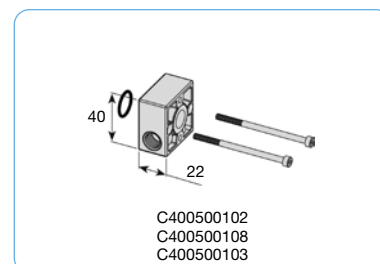
Verzweigungsplatte
